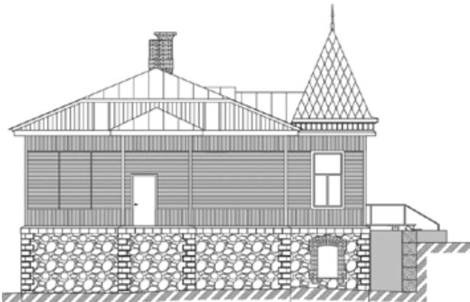
Северный фасад
