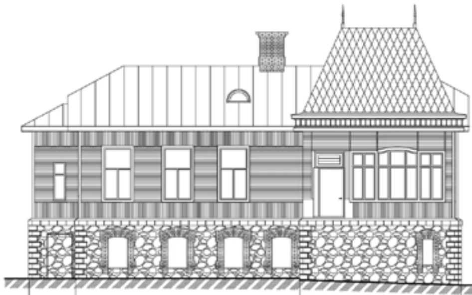
Северный фасад
