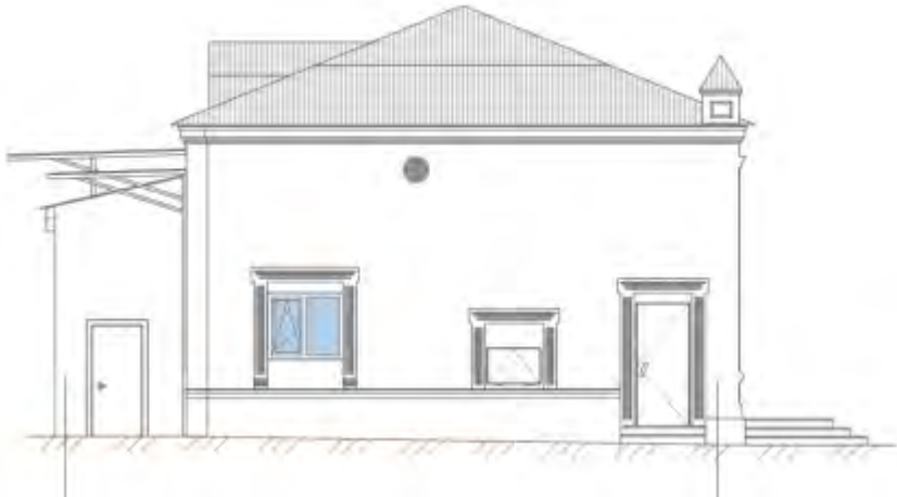
Восточный фасад
