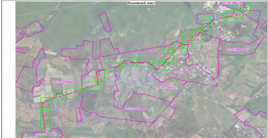
План границ охранной зоны объекта сети газораспределения (газопотребления) «Межпоселковый газопровод от ГРС Артем до ГГРП - 1 (п.Заводской) с отводом на ГГРП - 6, ГГРП - 7, ГГРП - 9»
