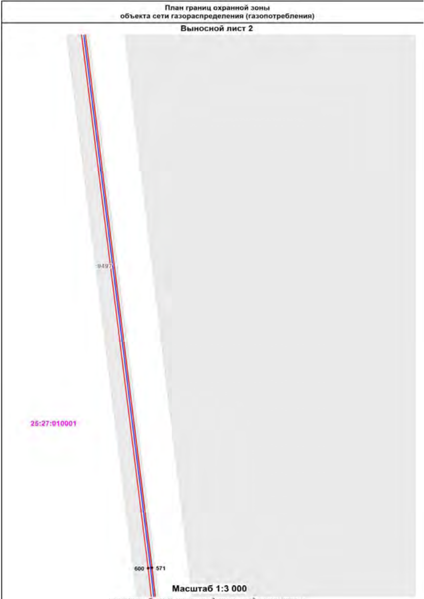
План границ охранной зоны объекта сети газораспределения (газопотребления) «Межпоселковый газопровод от ГРС Артем до ГГРП - 1 (п.Заводской) с отводом на ГГРП - 6, ГГРП - 7, ГГРП - 9»
